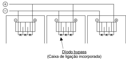
Figura 2. Paralelo para mais corrente
