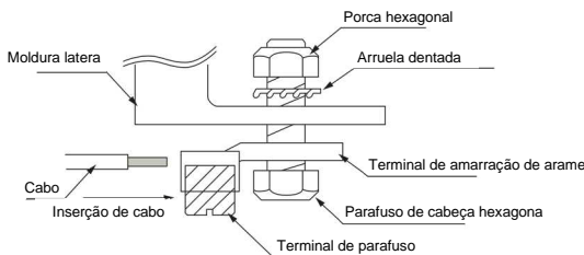
Figura 3: Exemplo de conexão de terra aceitável
