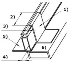
Figura 4. Requisitos de las sujeciones (abrazaderas)
