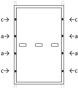
Fig. B2: Ubicación de los orificios para pernos
