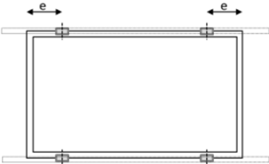
Fig. A2: Posição para prender na armação longa
