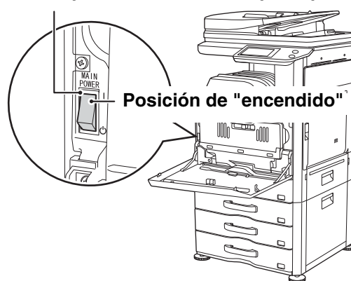
Interruptor de alimentación principal
