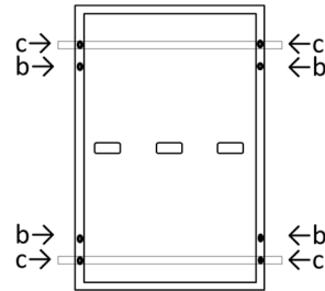
Fig. A3: Ubicación de los orificios para pernos
