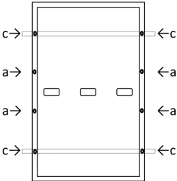
Fig. B1: Localização dos furos dos parafusos Trilhos de montagem perpendiculares à estrutura mais longa
