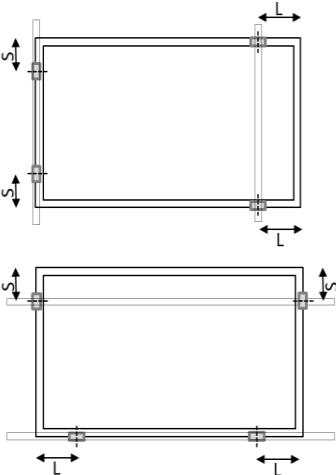
Fig. A3: Posición de las sujeciones en los marcos cortos y los marcos largos
