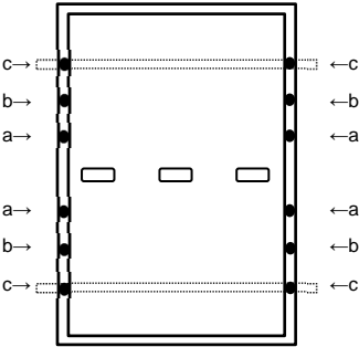
Fig. A3: Localização dos furos dos parafusos
