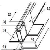
Figura 1. Requisitos de las sujeciones (abrazaderas)
