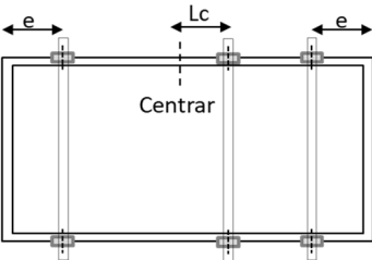
Fig. A1: Posición de las sujeciones en el marco largo
