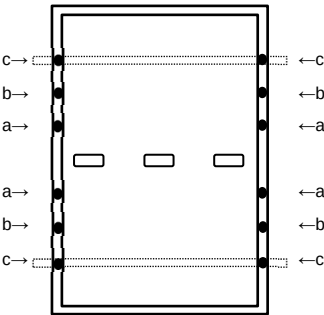
Fig. A3: Ubicación de los orificios para pernos
