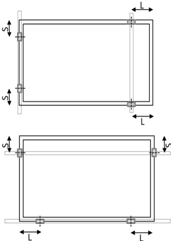
Fig. B: Posición de las sujeciones en los marcos corto y los marcos largos
