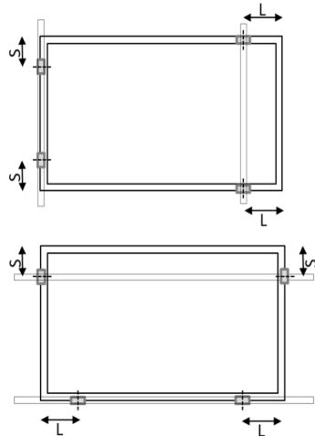
Fig. A3: Posición de las sujeciones en los marcos corto y los marcos largos
