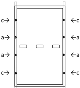
Fig. B2: Localização dos furos dos parafusos
