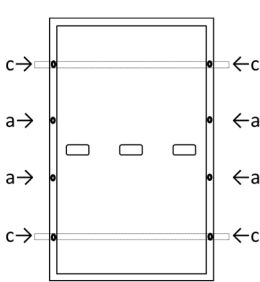
Fig. B1: Localização dos furos dos parafusos
