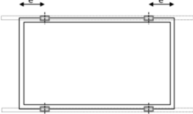
Fig. A2: Posición de las sujeciones en el marco corto Rieles de montaje paralelos al marco más largo
