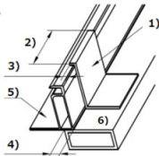
Figura 4. Requisitos das molas (grampos)
