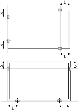
Fig. A3: Posição para prender nas armações longa e curta
