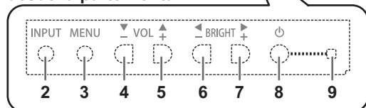
Botones posteriores vistos desde la parte frontal
