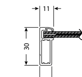
Seção transversal lateral curta do quadro
