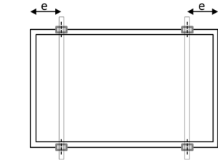
Fig. A1: Posición de las sujeciones en el marco largo
