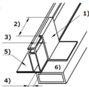
Figura 4. Requisitos das molas (grampos)
