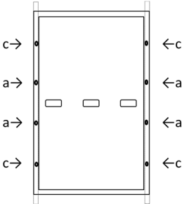
Fig. B2: Ubicación de los orificios para pernos Rieles de montaje paralelos al marco más largo
