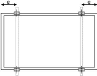
Fig. A1: Posición de las sujeciones en el marco largo Rieles de montaje perpendiculares al marco más largo
