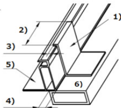
Figura 4. Requisitos de las sujeciones (abrazaderas)
