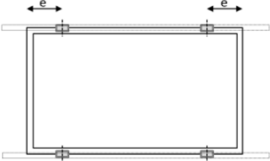
Fig. A2: Posición de las sujeciones en el marco corto Rieles de montaje paralelos al marco más largo
