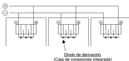
Figura 2. Paralelo para más corriente
