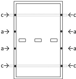
Fig. B1: Ubicación de los orificios para pernos Rieles de montaje perpendiculares al marco más largo
