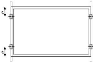
Fig. A2: Posição para prender na armação curta
