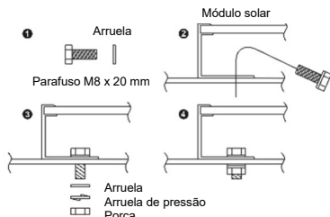
Figura 5. Os elementos do parafuso e porca
