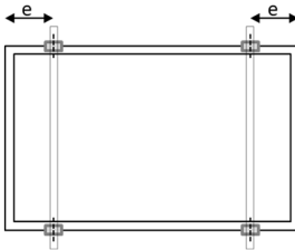
Fig. A1: Posición de las sujeciones en el marco largo
