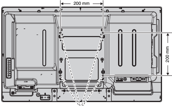
VESA Montaj Ara yüzü
