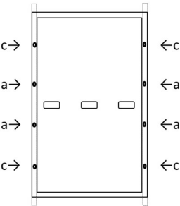
Fig. B2: Localização dos furos dos parafusos
