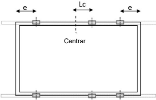
Fig. A2: Posição para prender na armação longa
